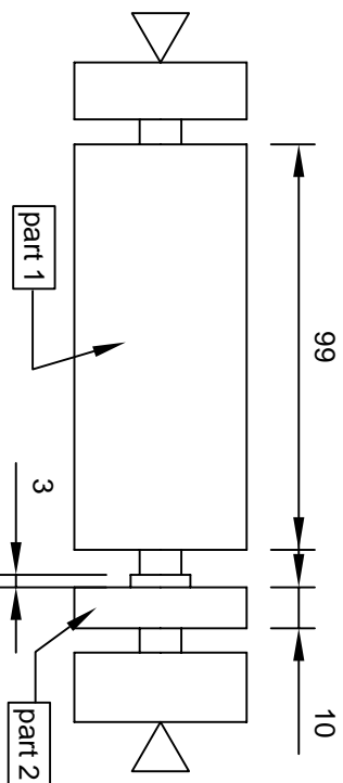
Turning blank setout
